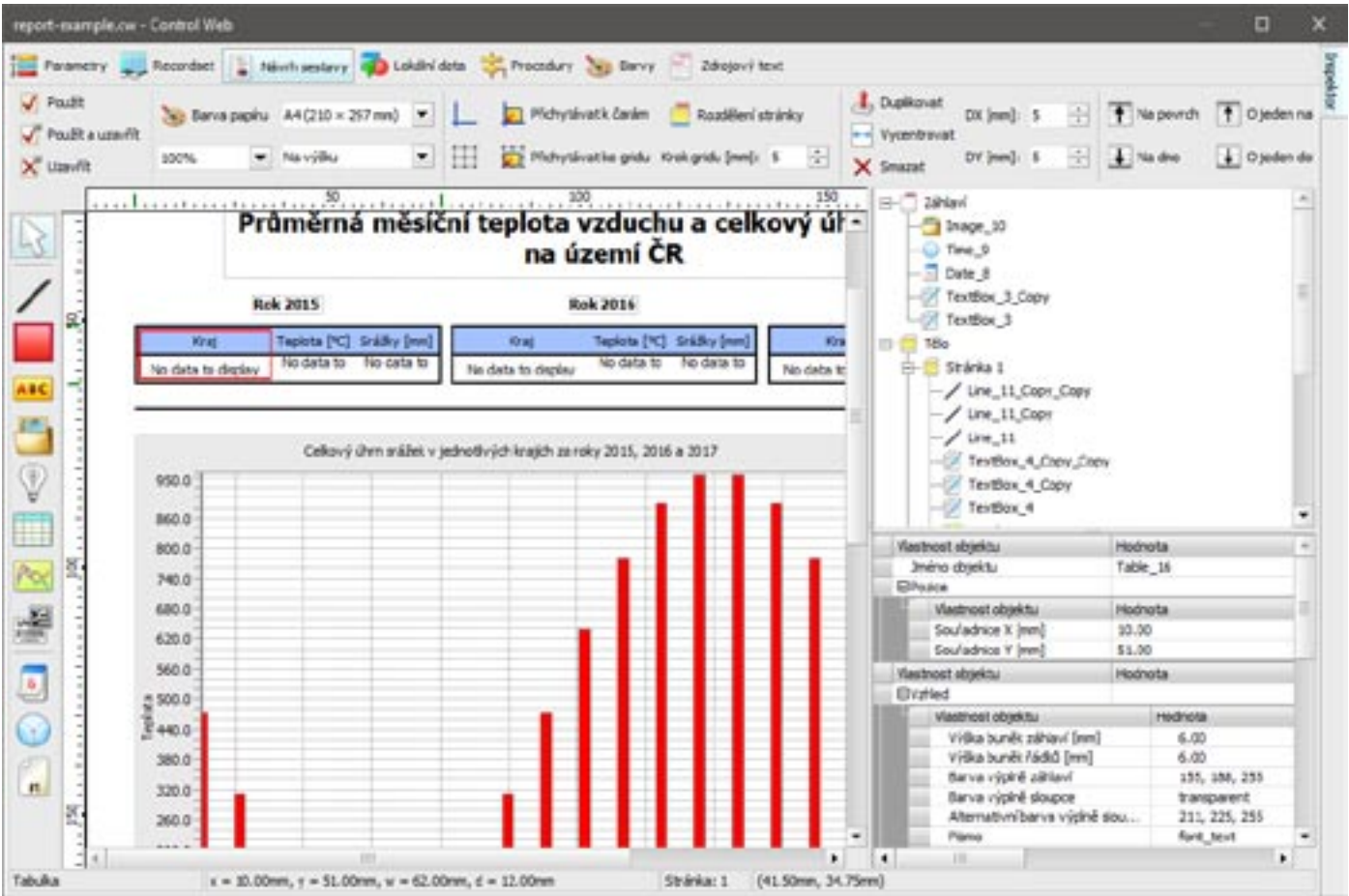
Editor sestavy v záložce inspektoru virtuálního přístroje.
